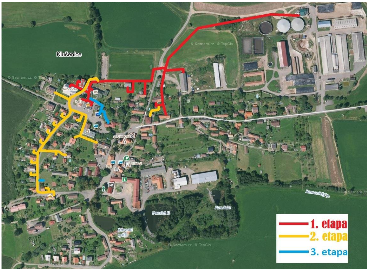
Plánek všech tří etap výstavby teplovodu
